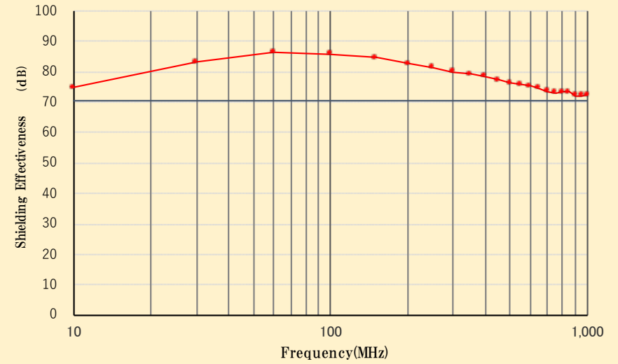
シールド効果（電界）：UC-30H
