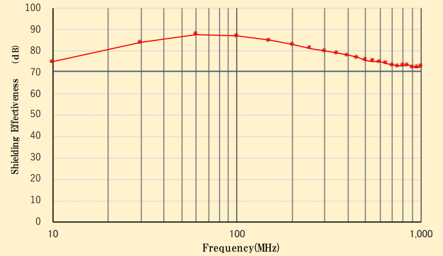
シールド効果（電界）：UC-20F
