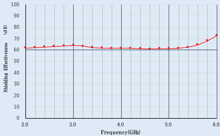
シールド効果（電磁界）：UC-10K
