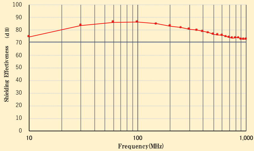
シールド効果（電界）：UC-10K
